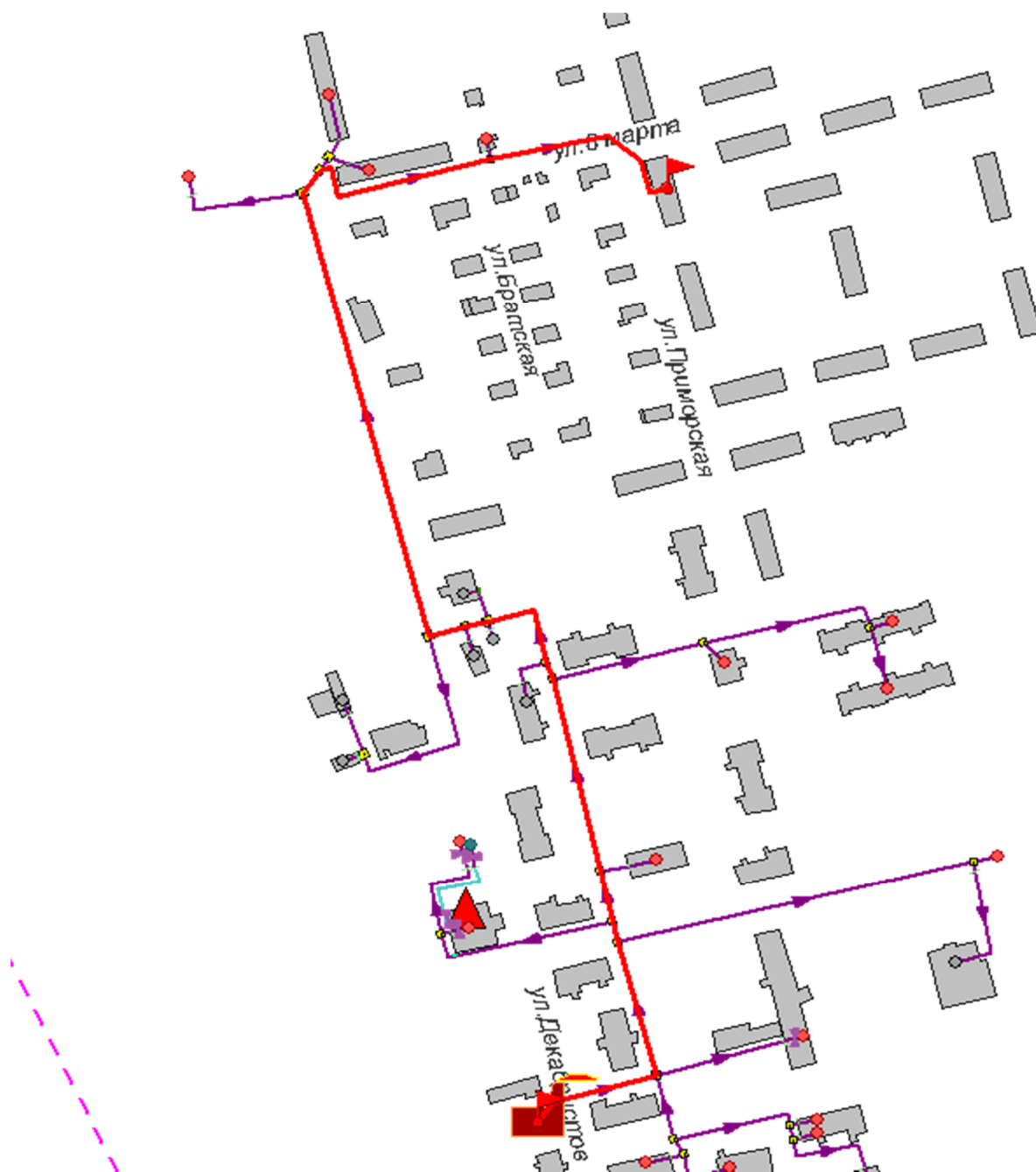
Рисунок 24.3 -Расчетный путь теплоносителя от котельной до Приморская,16
