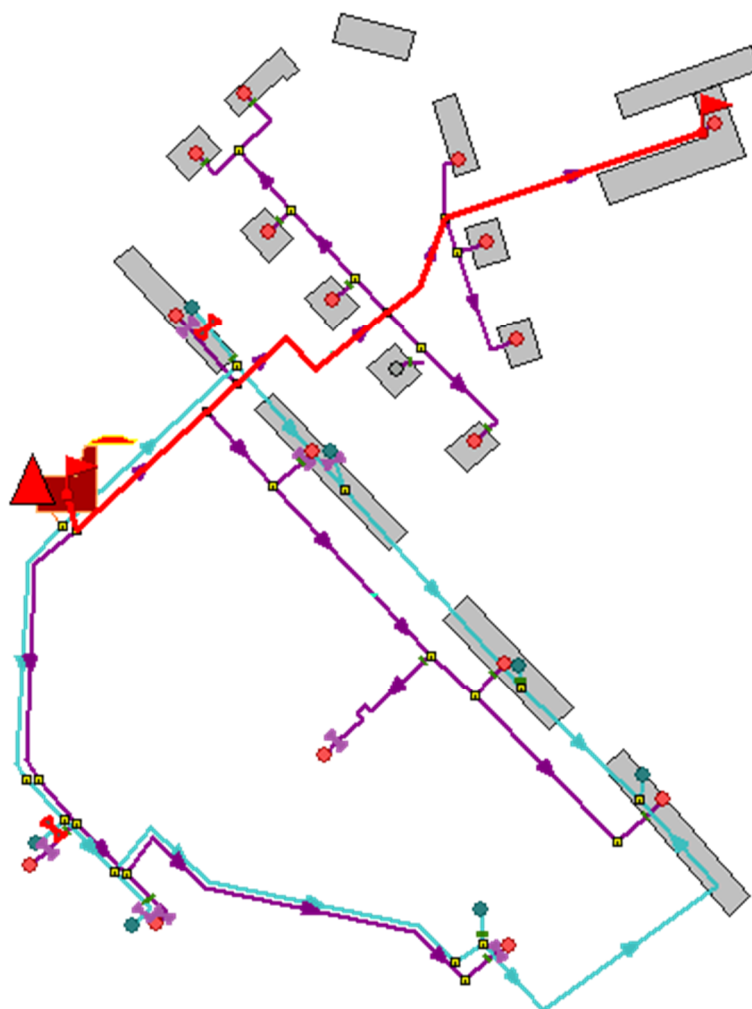
Рисунок 21.1 -Расчетный путь теплоносителя котельной до Лахтинское шоссе,135
