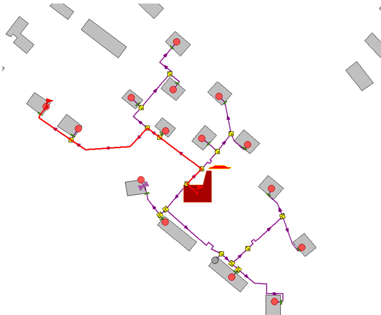
Рисунок 6.1 -Расчетный путь теплоносителя котельной до Дрейера, 15 к.3
