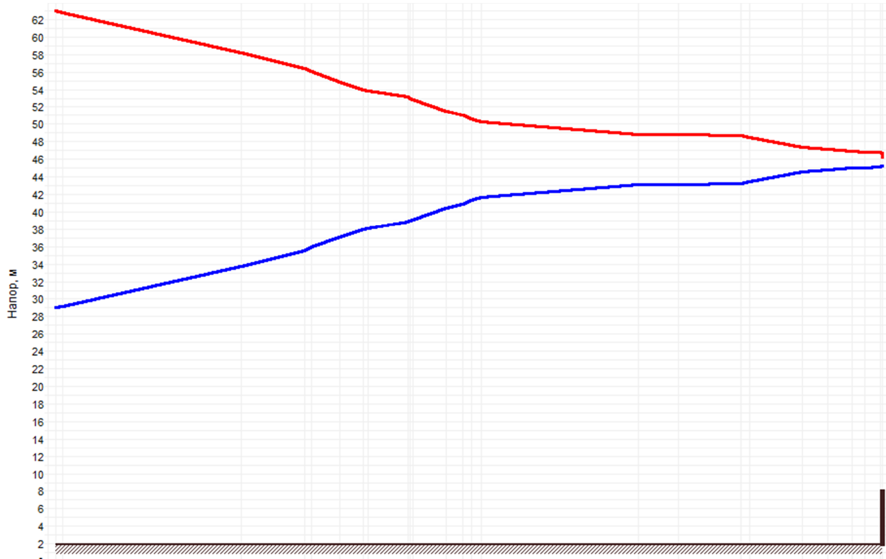
Рисунок 10.2 –График гидравлических режимов рассматриваемого теплопровода
