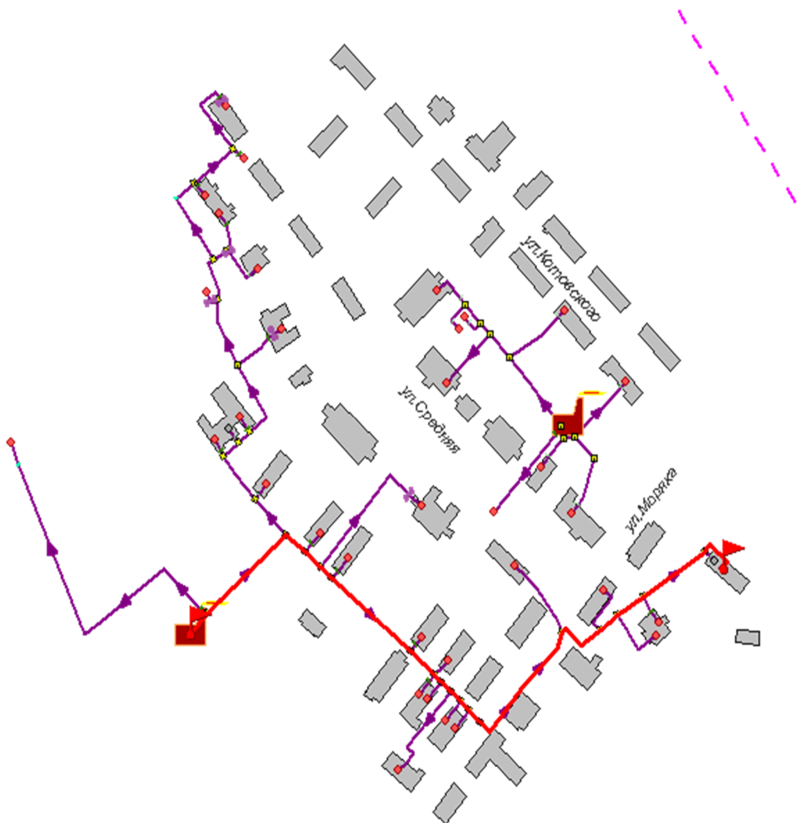
Рисунок 25.1 -Расчетный путь теплоносителя котельной до Моряка,1
