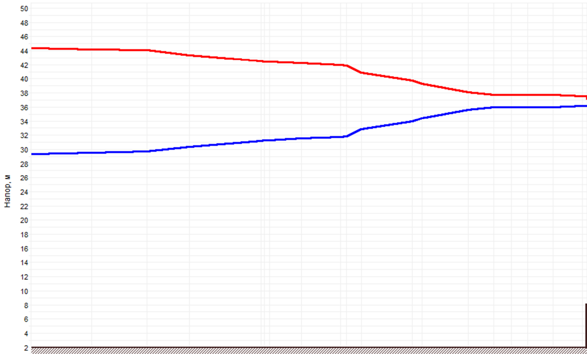
Рисунок 33.2 –График гидравлических режимов рассматриваемого теплопровода
