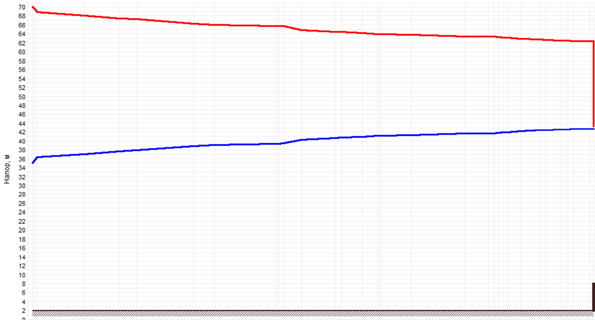
Рисунок 34.4 –График гидравлических режимов рассматриваемого теплопровода
