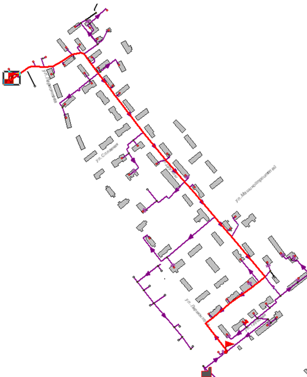
Рисунок 13.1 -Расчетный путь теплоносителя котельной до Лермонтова 23, стр.20
