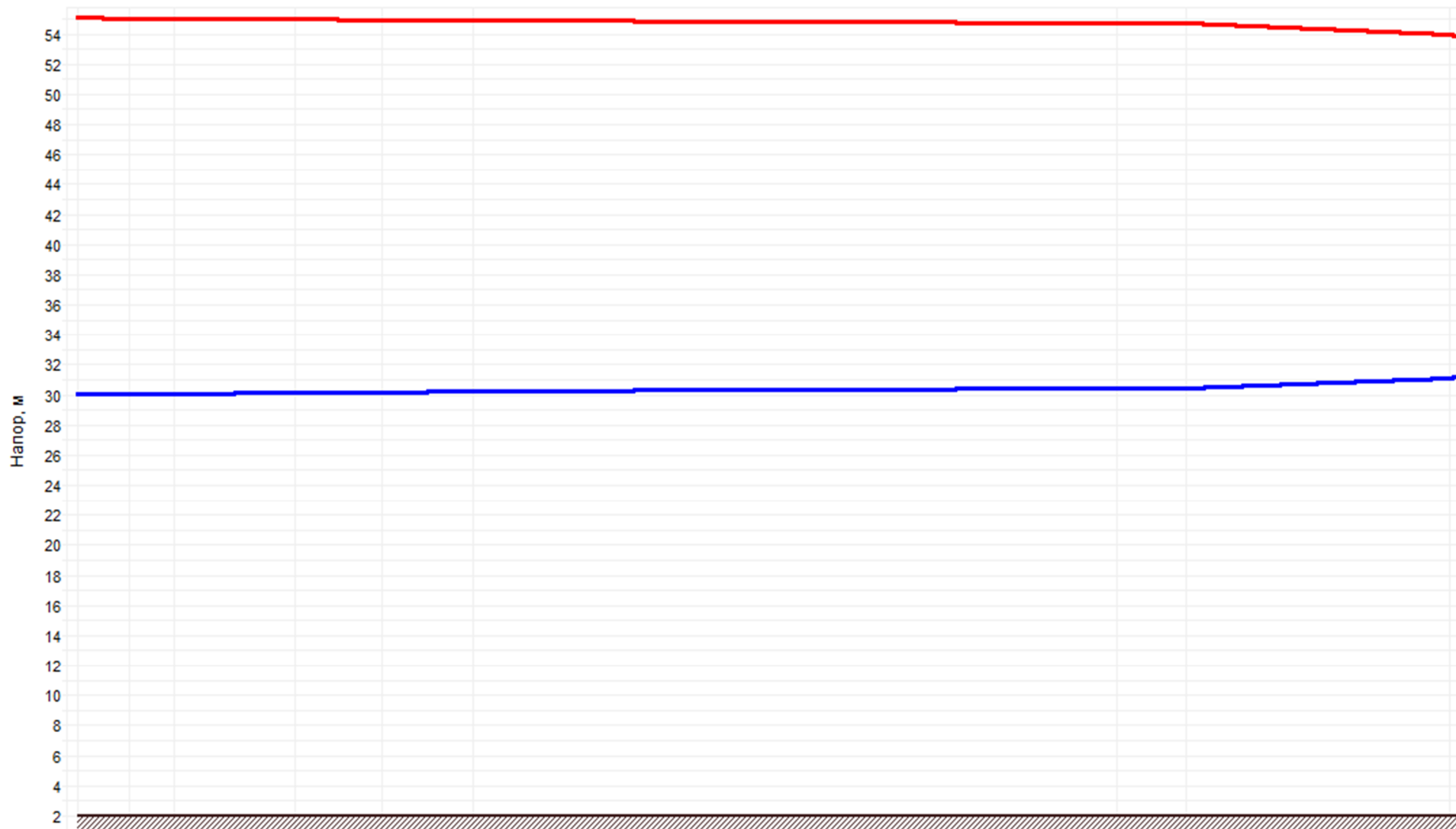
Рисунок 9.2 –График гидравлических режимов рассматриваемого теплопровода
