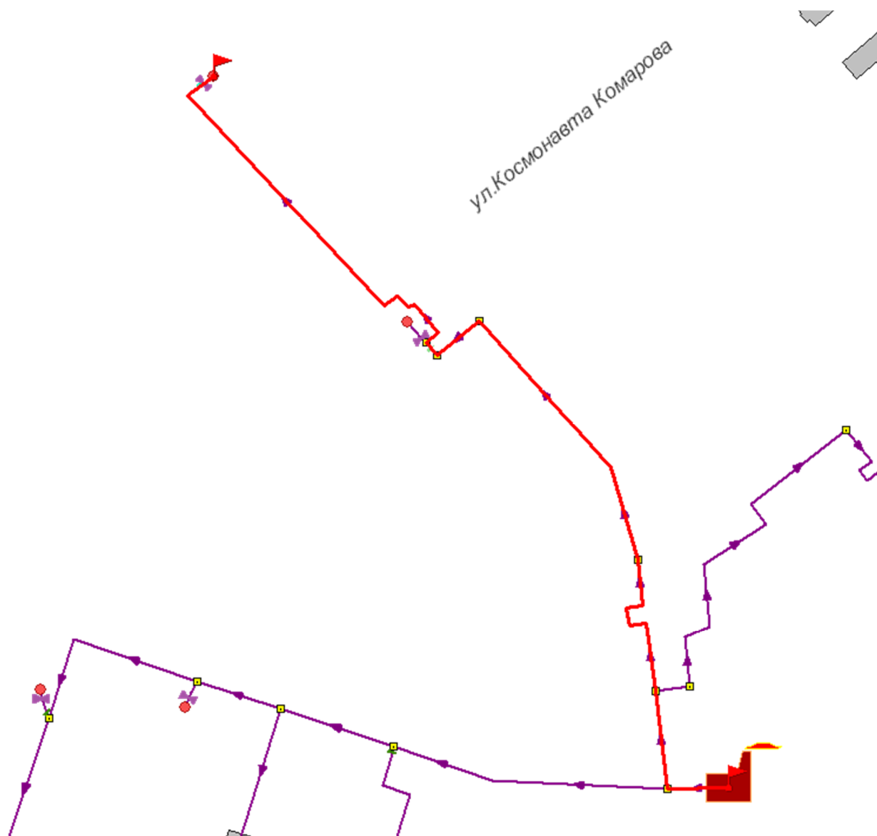
Рисунок 35.3 -Расчетный путь теплоносителя от котельной до Комарова, 14
