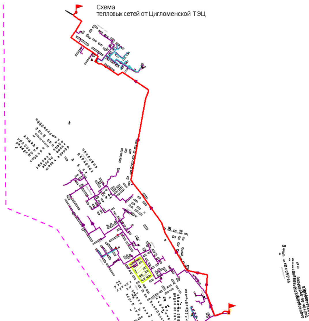
Рисунок 2.1 -Расчетный путь теплоносителя от Цигломенской ТЭС до кирпичного завода
