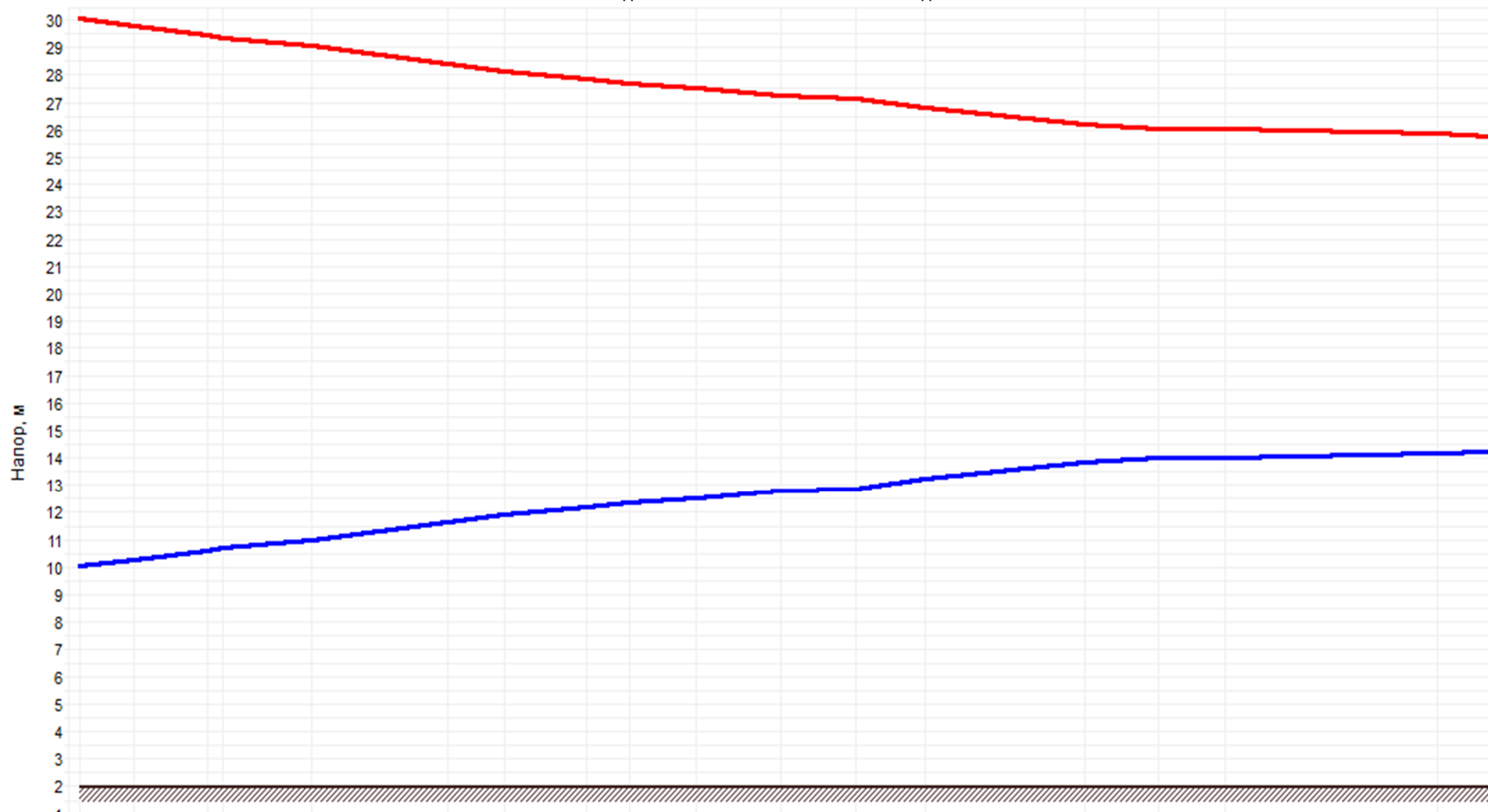
Рисунок 29.2 –График гидравлических режимов рассматриваемого теплопровода
