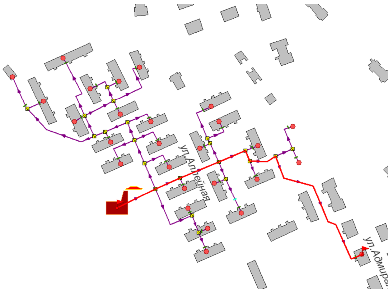
Рисунок 12.1 -Расчетный путь теплоносителя котельной доАдм. Макарова, 15
