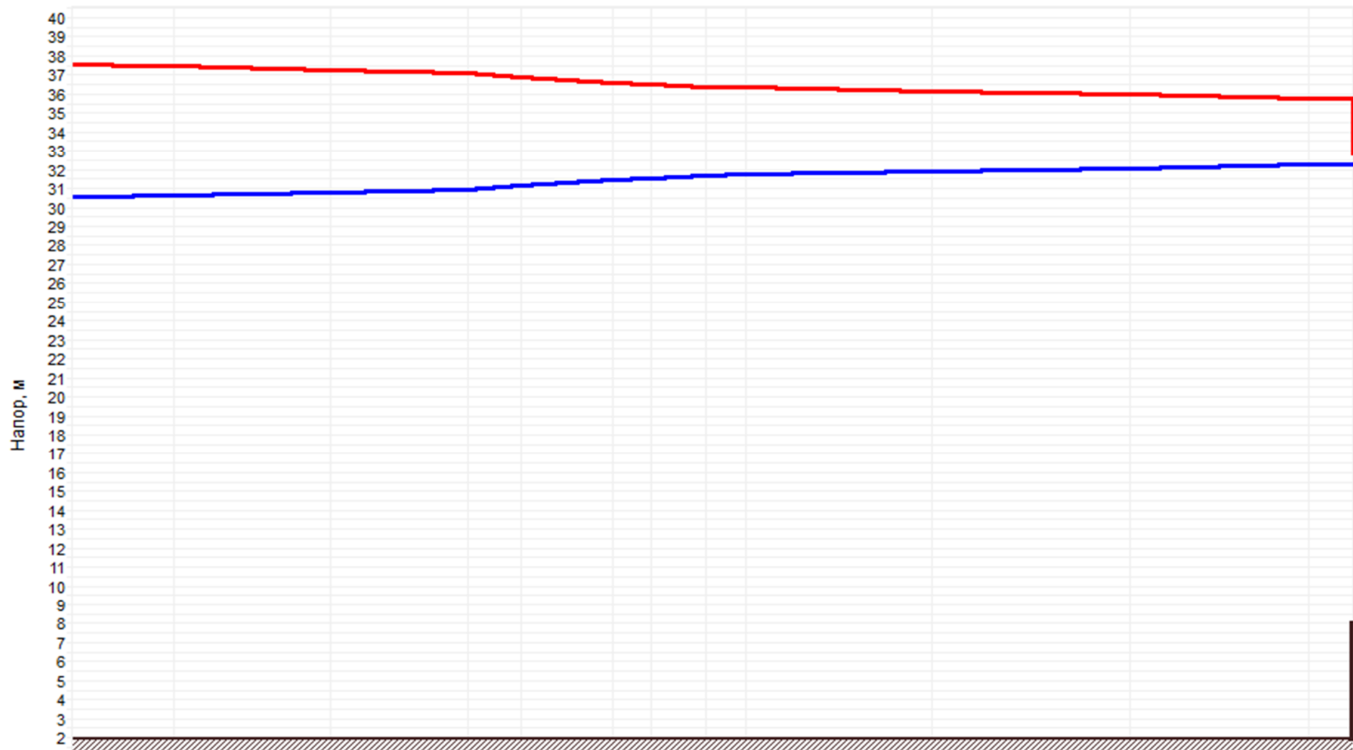
Рисунок 19.4 –График гидравлических режимов рассматриваемого теплопровода
