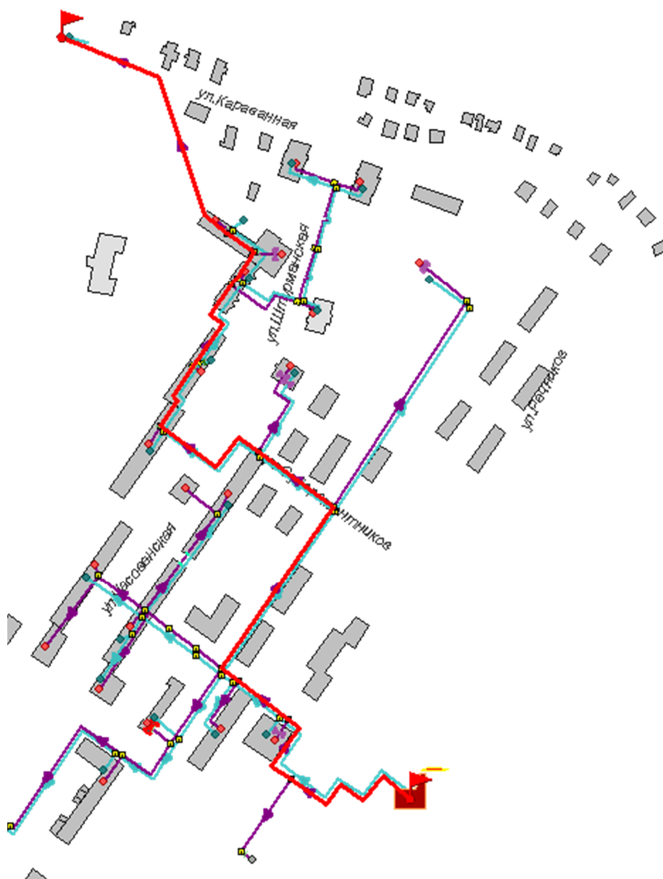
Рисунок 15.3 -Расчетный путь теплоносителя от котельной до очистных сооружений
