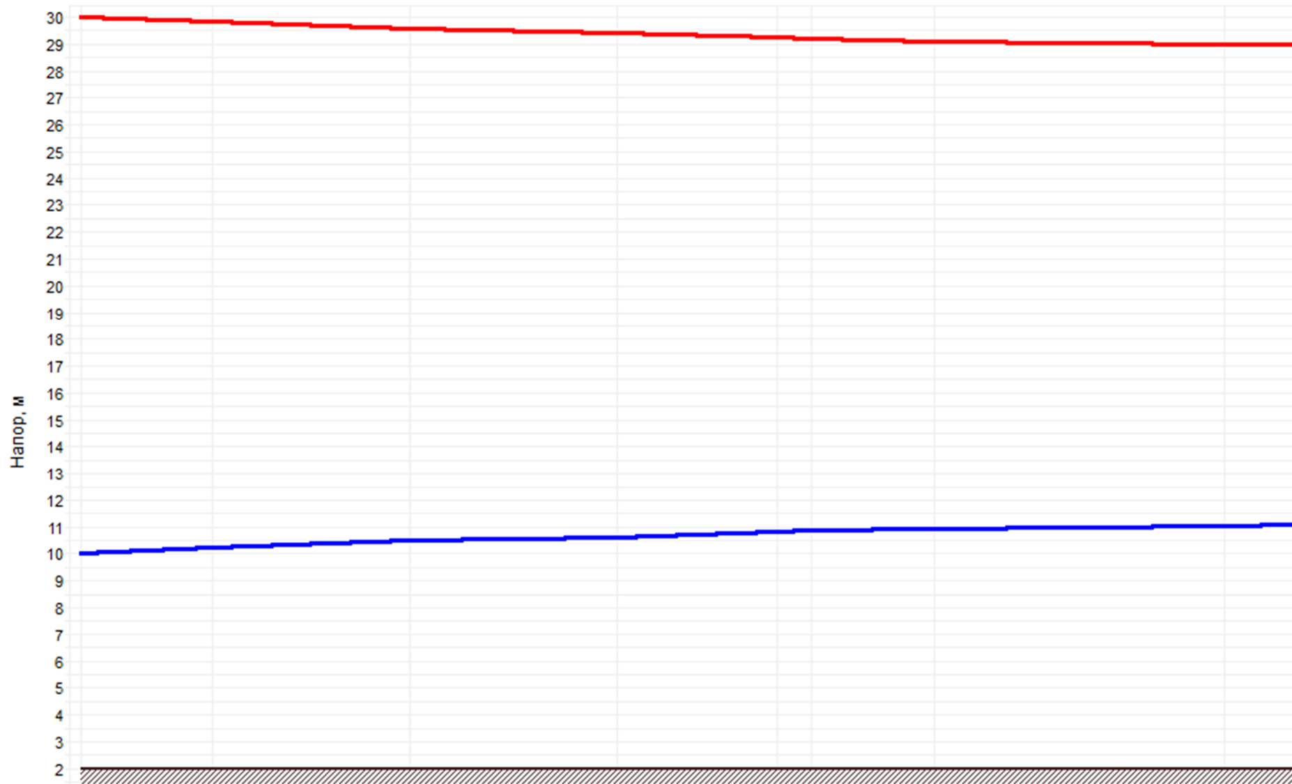
Рисунок 17.2 –График гидравлических режимов рассматриваемого теплопровода
