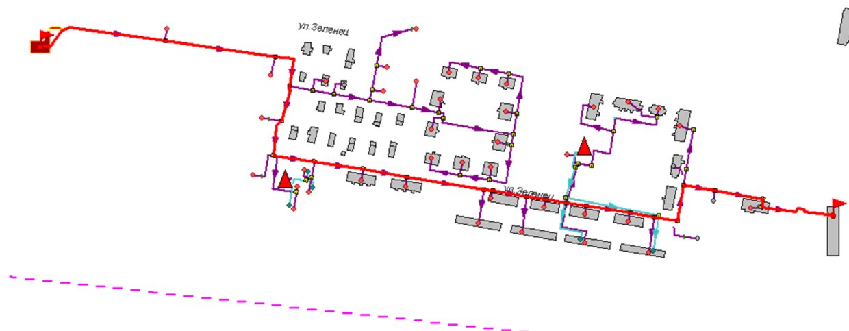
Рисунок 4.1 -Расчетный путь теплоносителя котельной до Зеленец, 1 к.1
