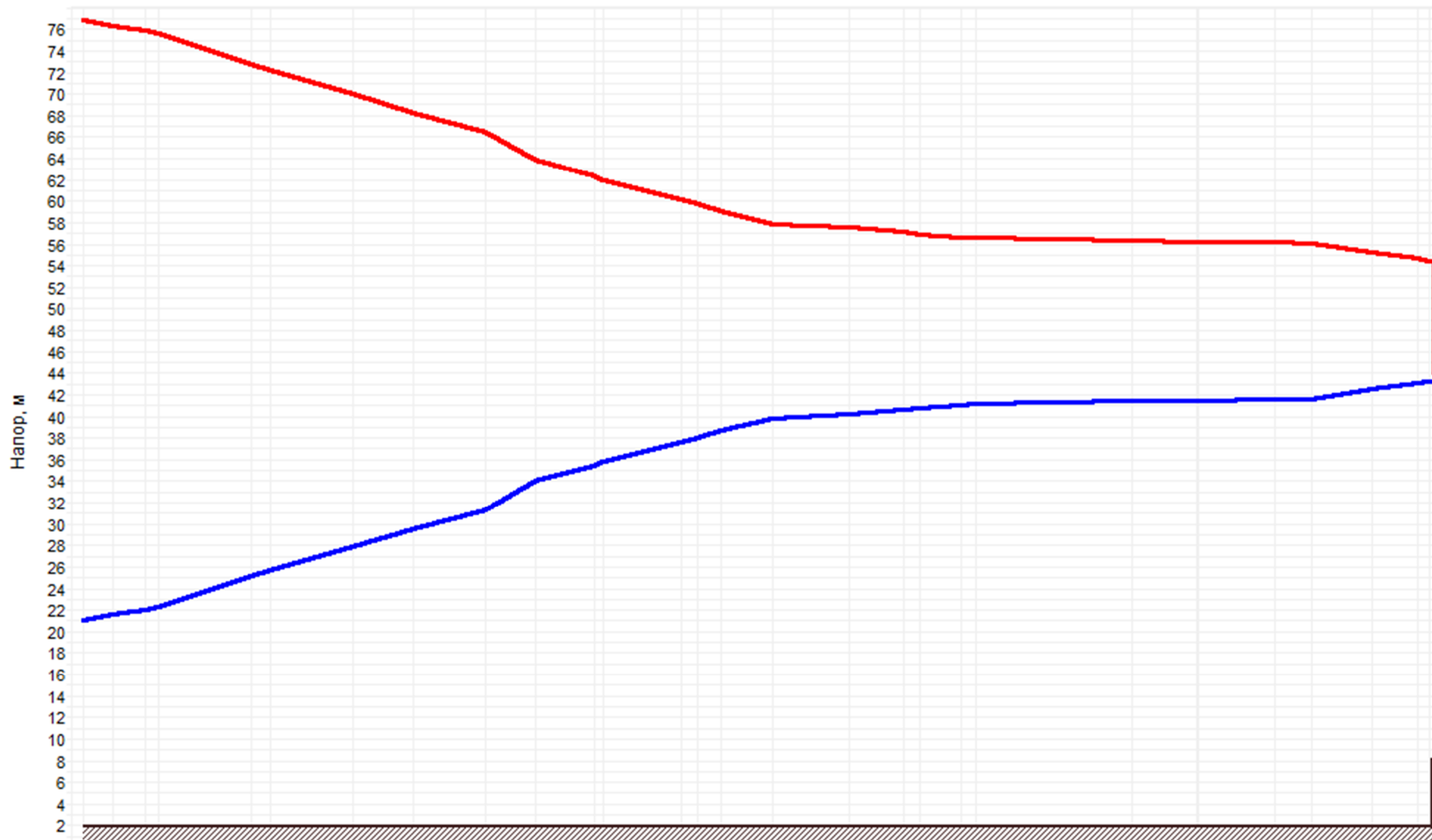
Рисунок 2.4 –График гидравлических режимов рассматриваемого теплопровода
