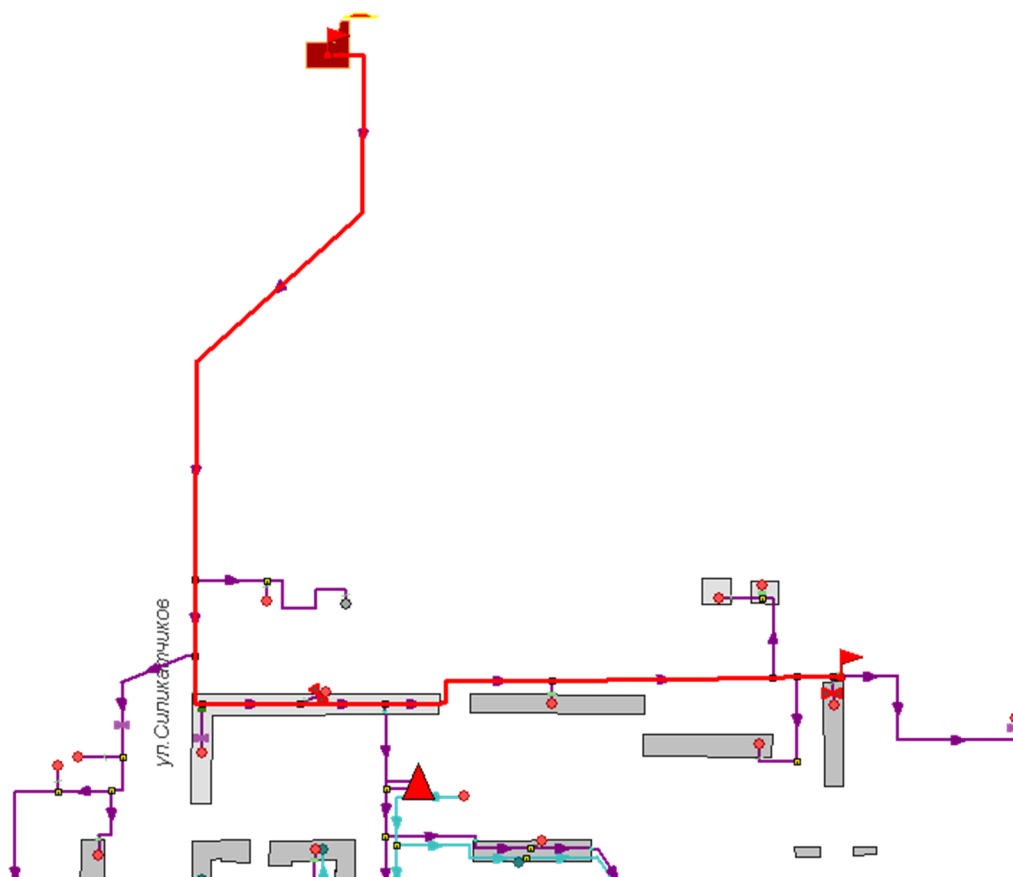
Рисунок 14.1 -Расчетный путь теплоносителя котельной до Лермонтова 23, стр.20
