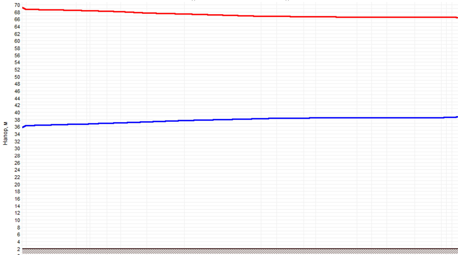
Рисунок 34.2 –График гидравлических режимов рассматриваемого теплопровода
