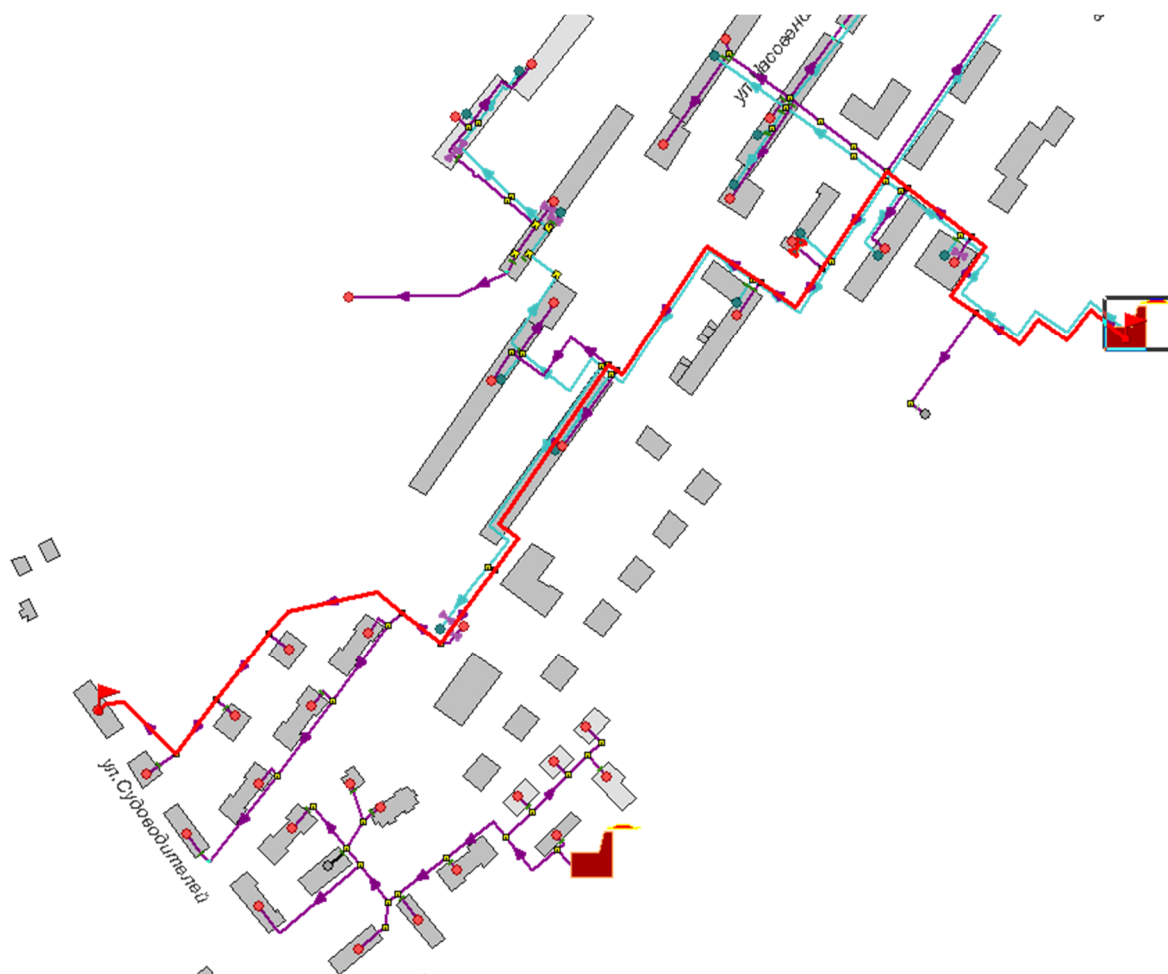
Рисунок 15.1 -Расчетный путь теплоносителя от котельной до Сив. Дивизии, 1
