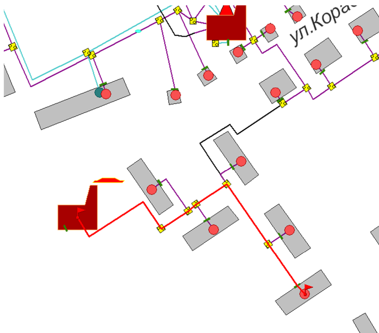
Рисунок 30.1 -Расчетный путь теплоносителя котельной до Кучина, 1
