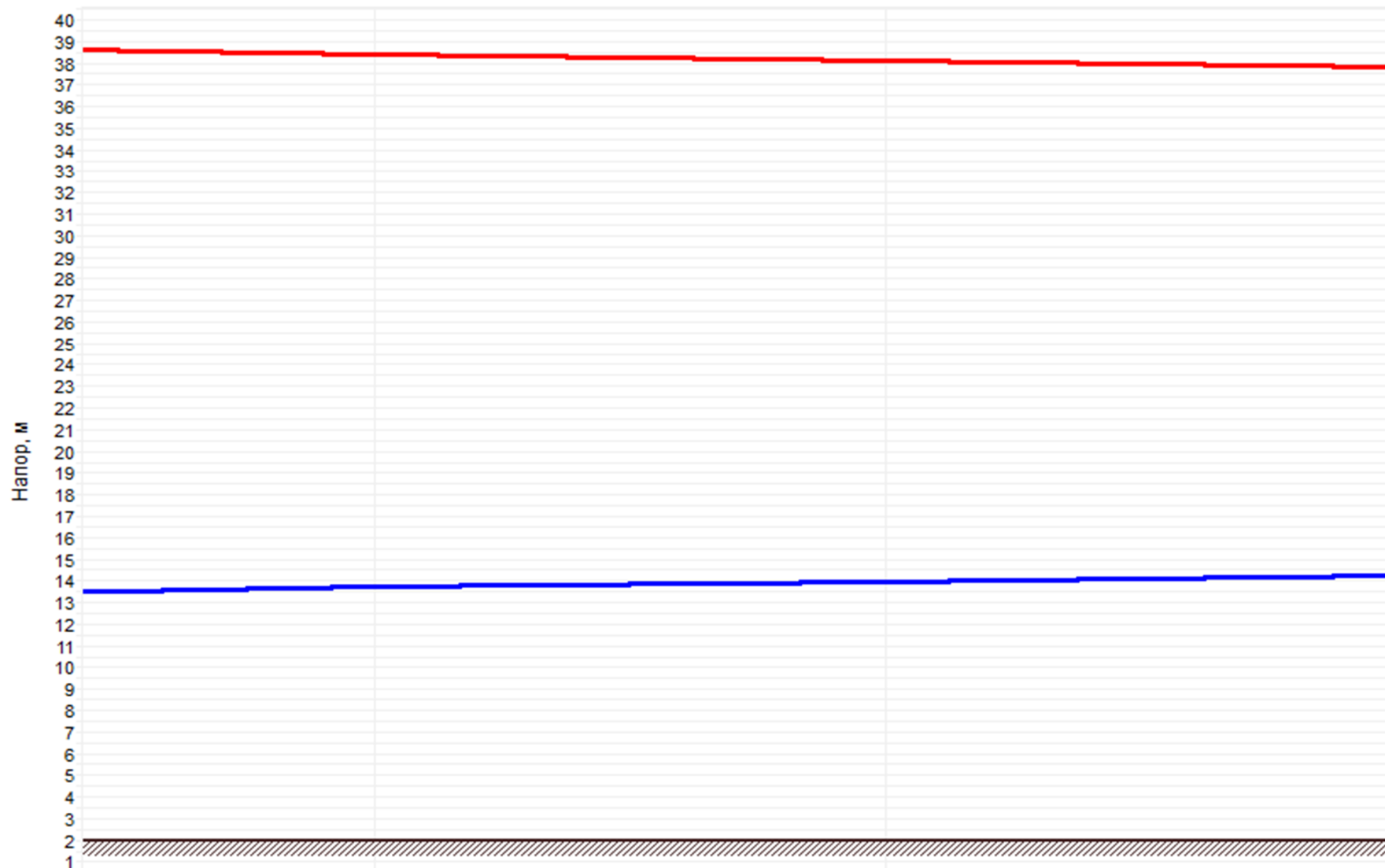
Рисунок 21.2 –График гидравлических режимов рассматриваемого теплопровода
