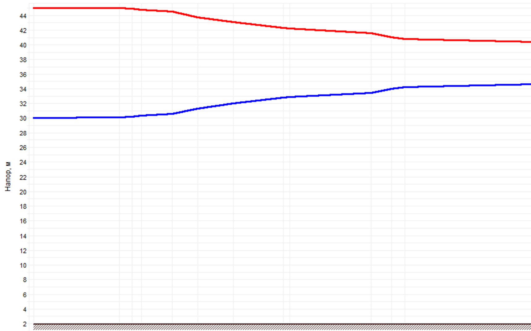
Рисунок 31.4 –График гидравлических режимов рассматриваемого теплопровода
