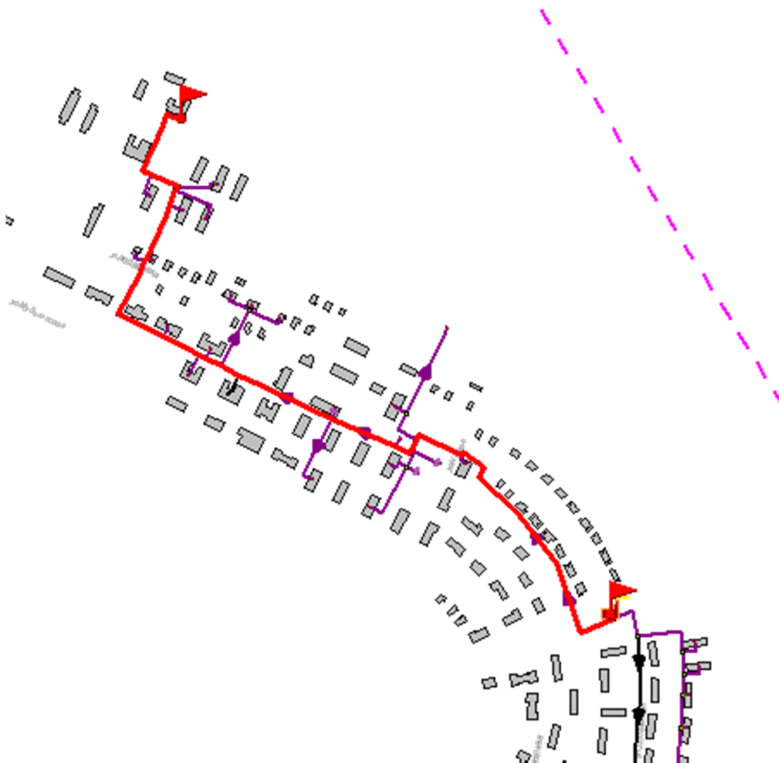
Рисунок 36.1 -Расчетный путь теплоносителя котельной до Карская,15, амбулатория 29л/з
