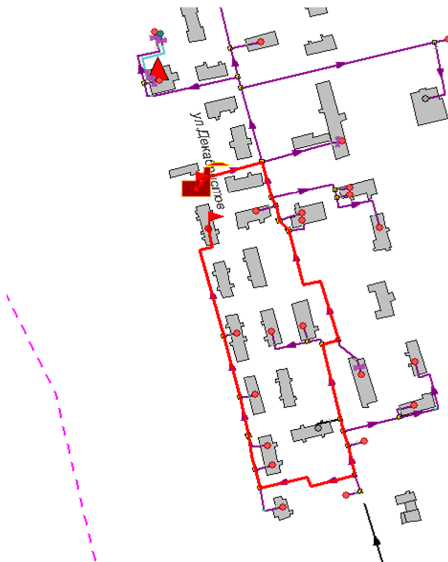
Рисунок 24.1 -Расчетный путь теплоносителя от котельной до Декабристов,15
