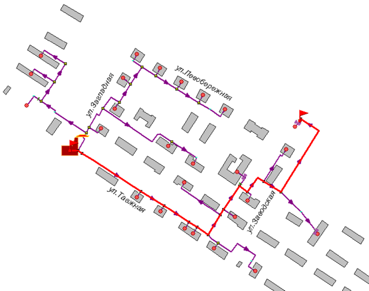
Рисунок 22.1 -Расчетный путь теплоносителя котельной до Турдеево, ПЧ-70
