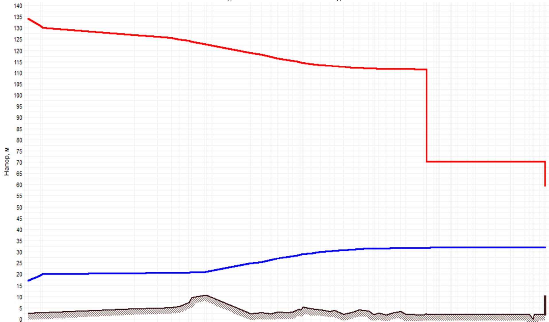
Рисунок 1.6 –График гидравлических режимов рассматриваемого теплопровода
