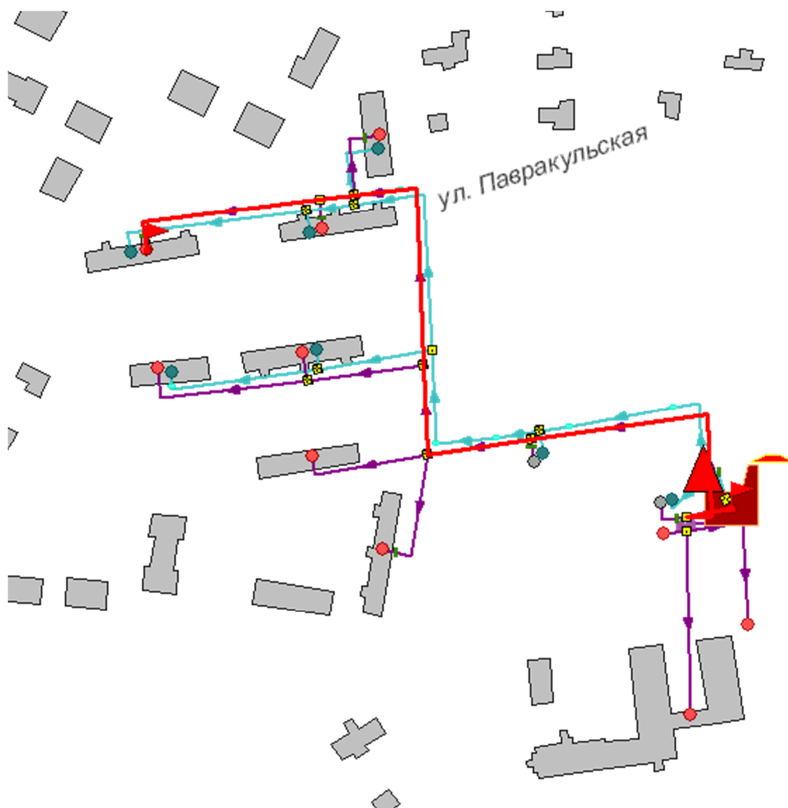
Рисунок 32.1 -Расчетный путь теплоносителя котельной до Победы,12,к.2
