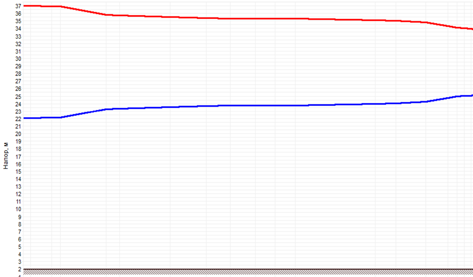
Рисунок 3.2 –График гидравлических режимов рассматриваемого теплопровода
