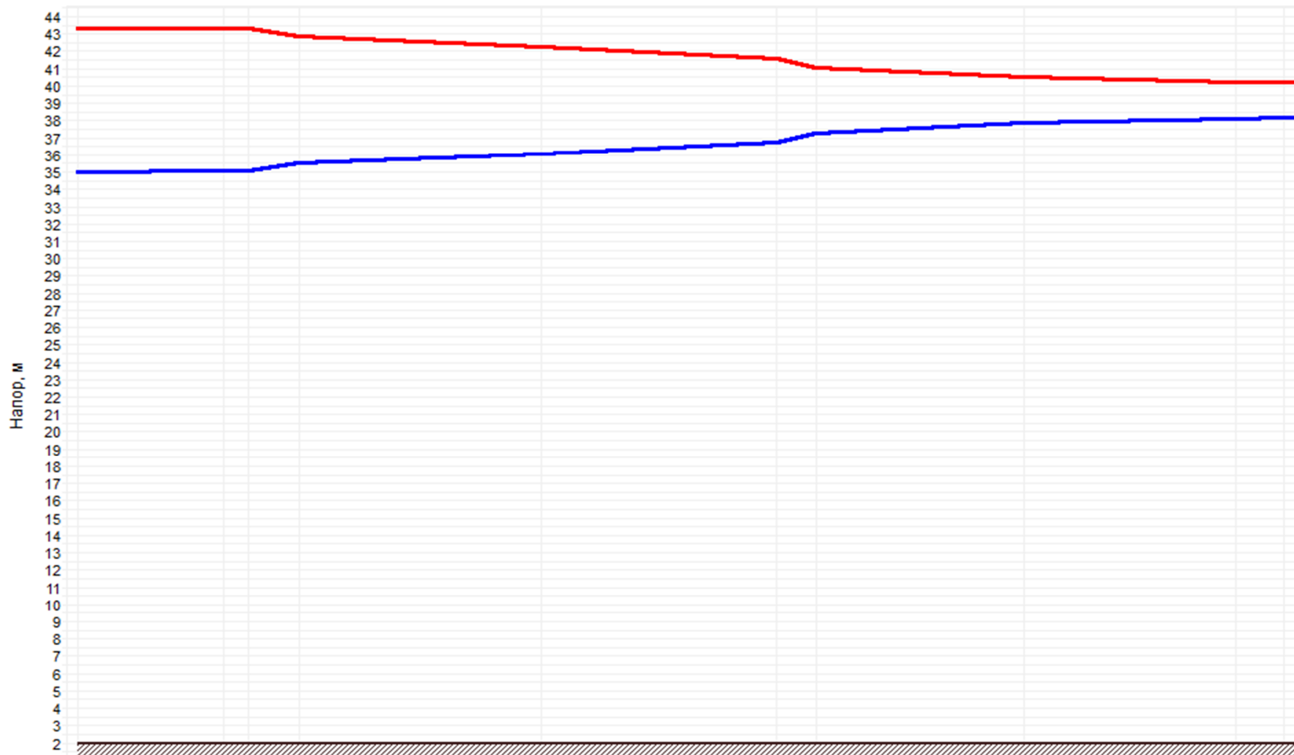
Рисунок 20.2 –График гидравлических режимов рассматриваемого теплопровода
