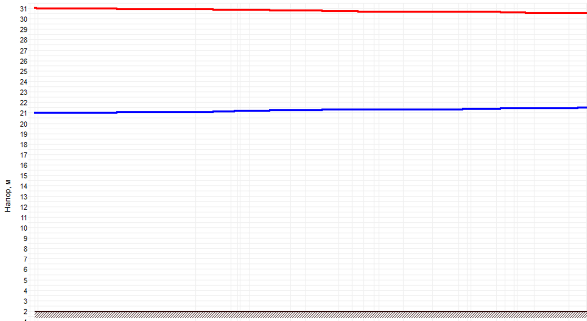
Рисунок 36.2 –График гидравлических режимов рассматриваемого теплопровода
