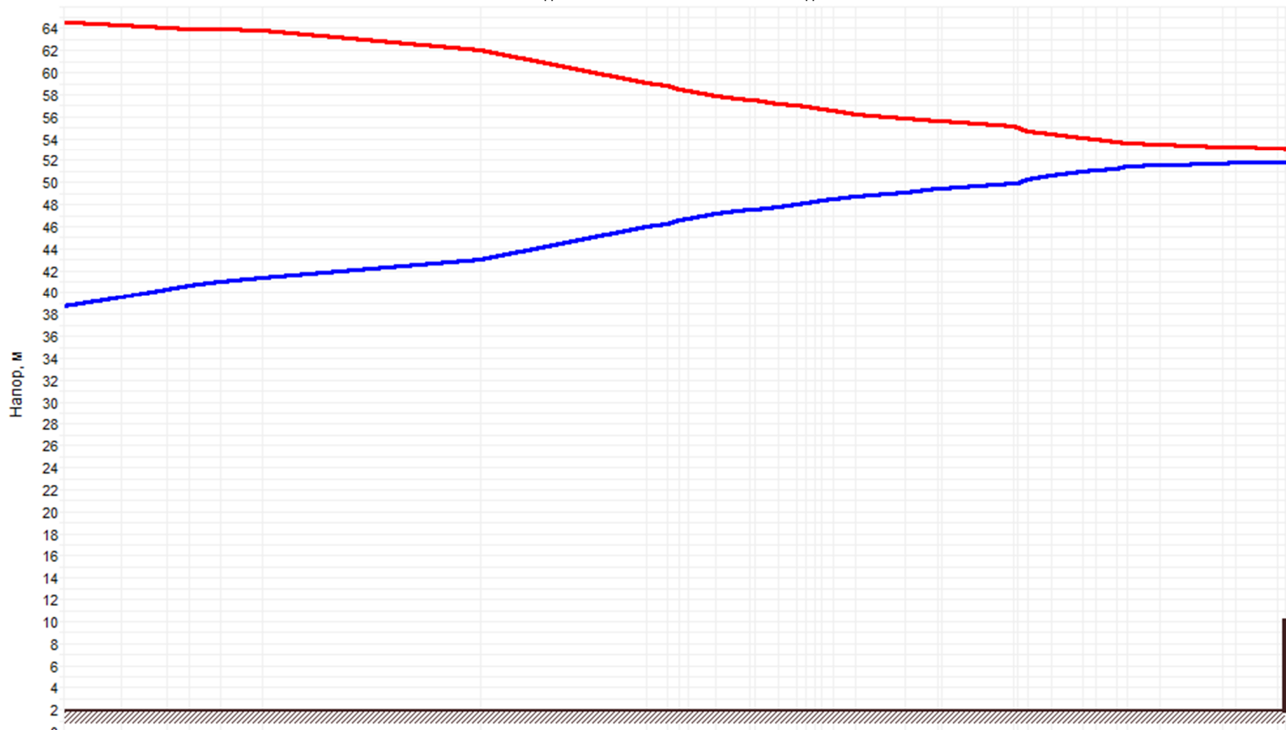
Рисунок 26.2 –График гидравлических режимов рассматриваемого теплопровода
