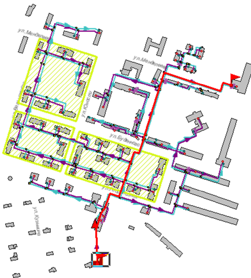
Рисунок 31.3 -Расчетный путь теплоносителя от котельной до Менделеева,19
