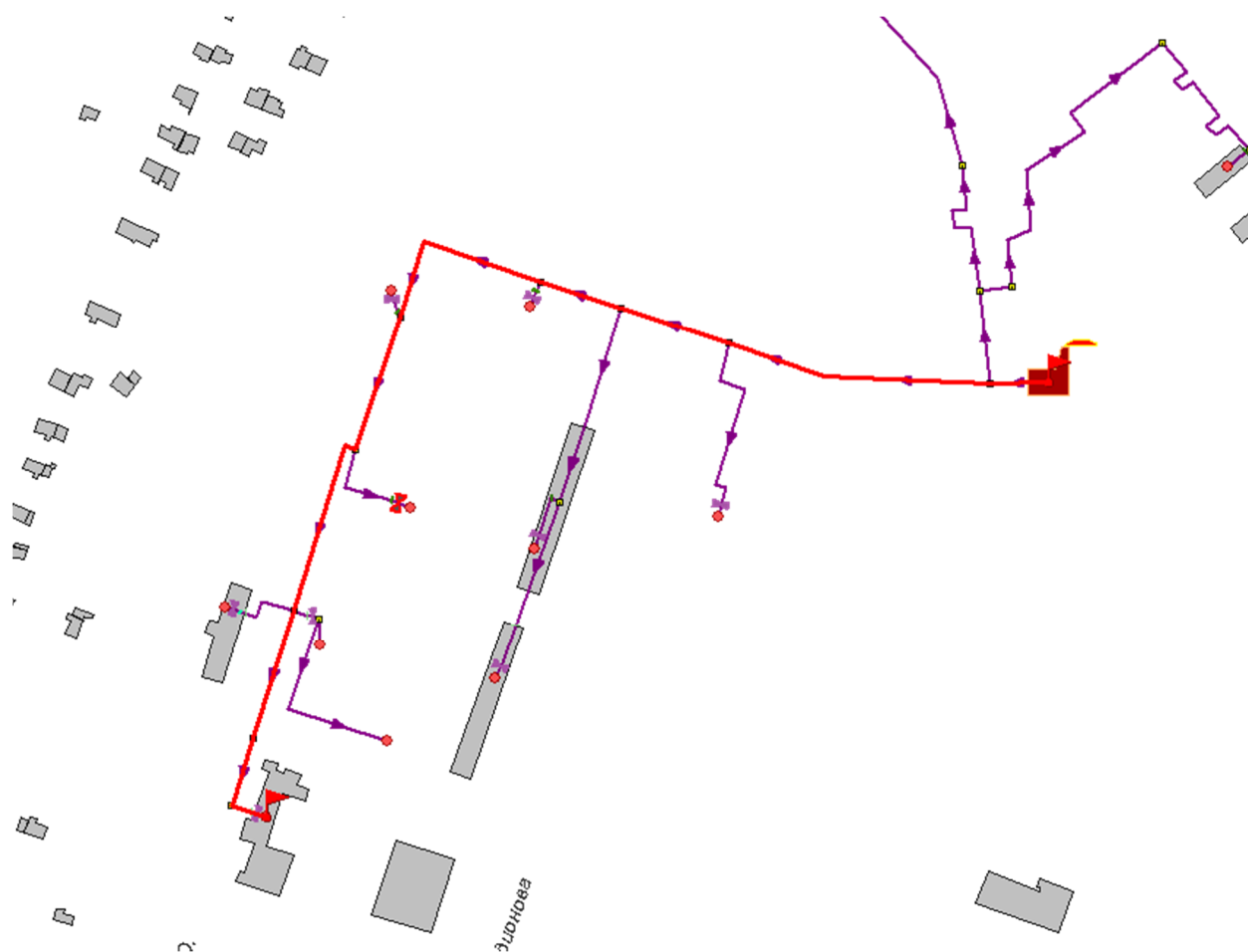
Рисунок 35.1 -Расчетный путь теплоносителя от котельной до Капитана Храмцова,5а
