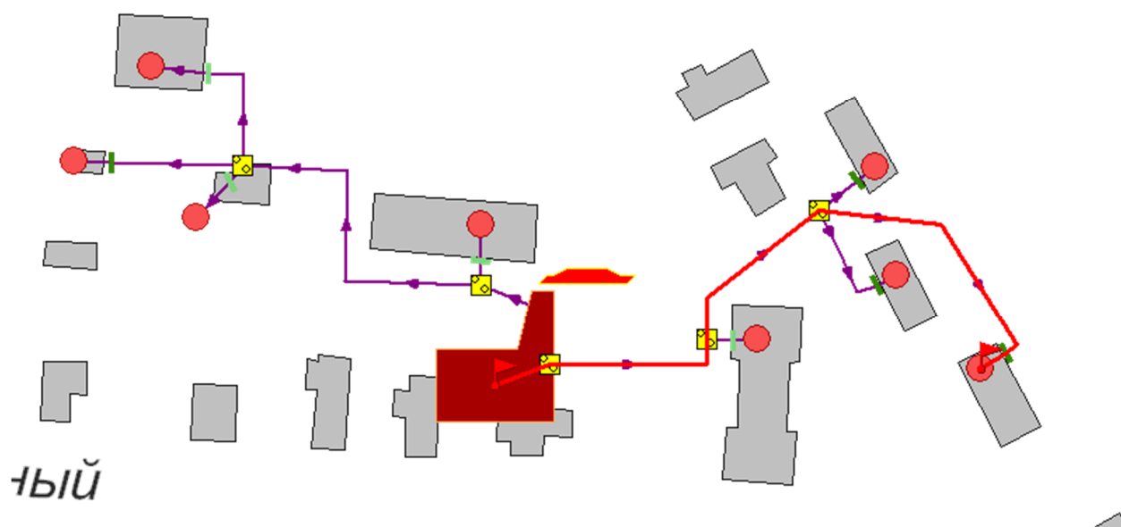
Рисунок 7.1 -Расчетный путь теплоносителя котельной до Северный, 12
