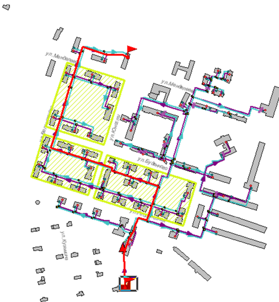
Рисунок 31.1 -Расчетный путь теплоносителя от котельной до Юности,2
