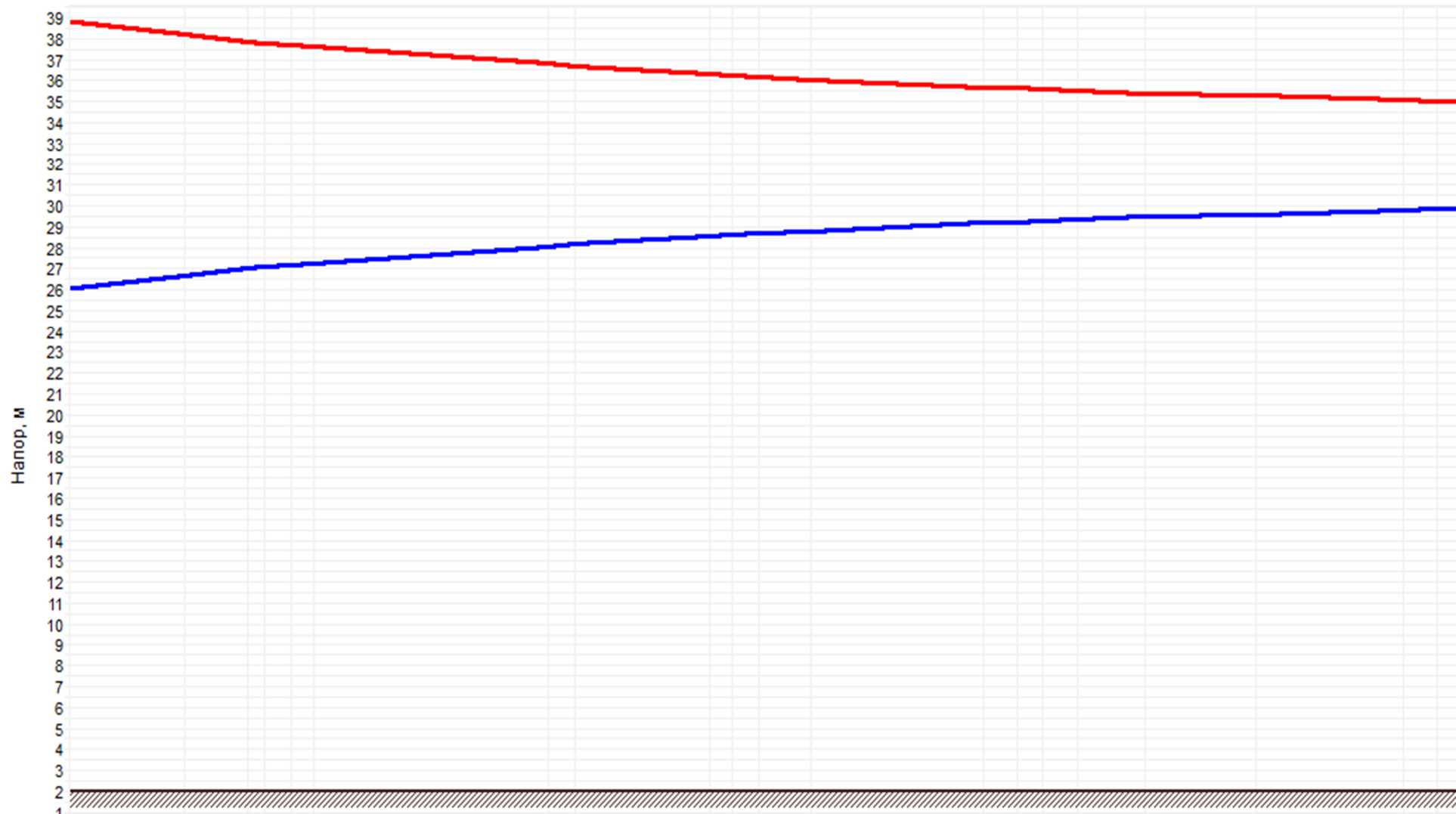
Рисунок 24.2 –График гидравлических режимов рассматриваемого теплопровода
