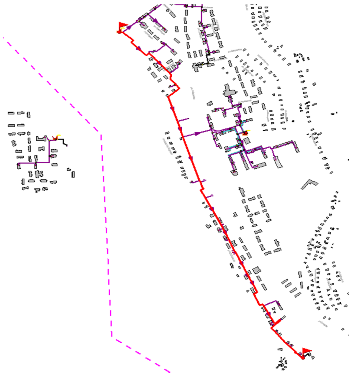
Рисунок 34.3 -Расчетный путь теплоносителя от котельной до ТСЖ «Зеленый квартал»
