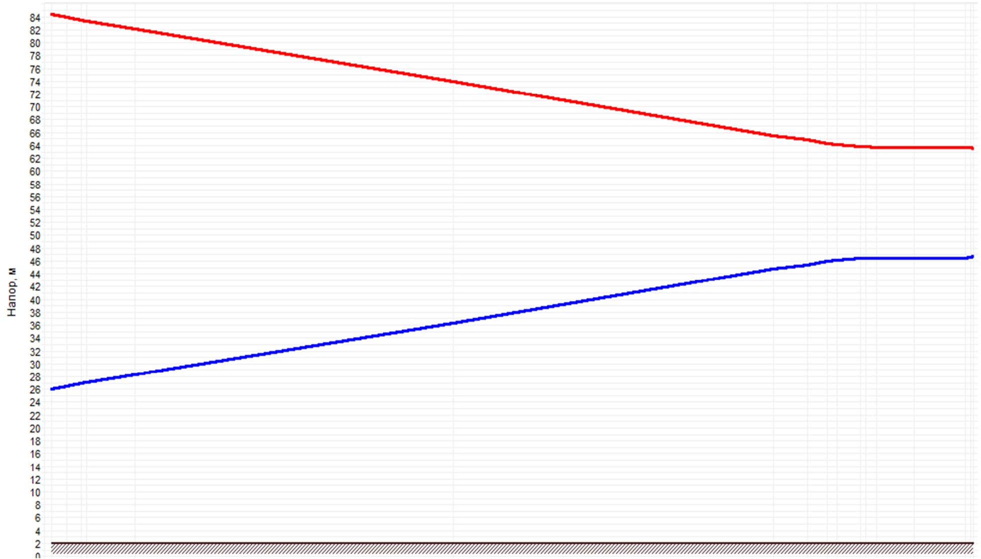
Рисунок 2.2 –График гидравлических режимов рассматриваемого теплопровода
