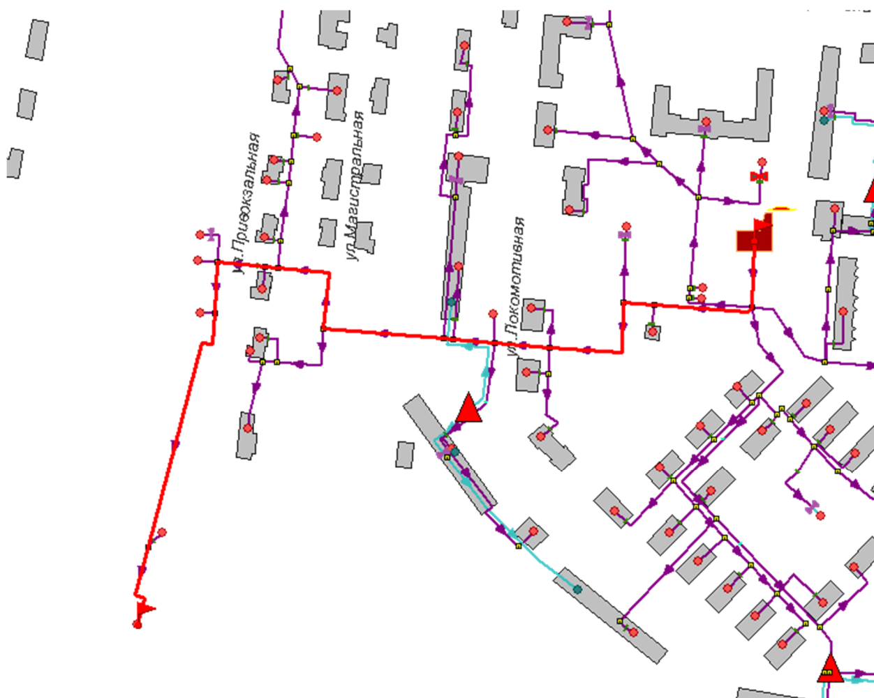
Рисунок 19.1 -Расчетный путь теплоносителя от котельной до Привокзальная, 19
