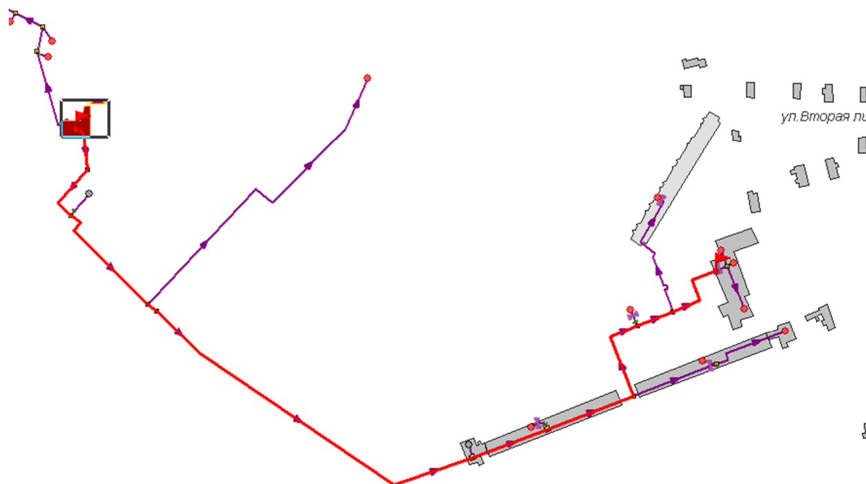
Рисунок 18.1 -Расчетный путь теплоносителя котельной до 2-я линия,9
