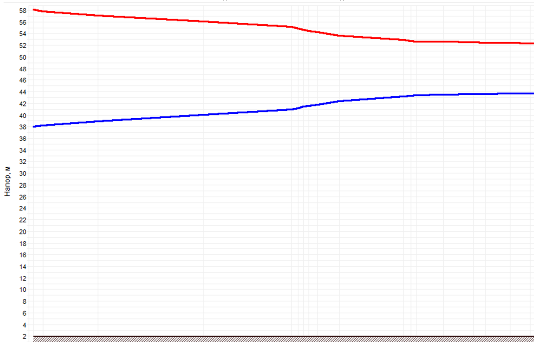
Рисунок 16.2 –График гидравлических режимов рассматриваемого теплопровода
